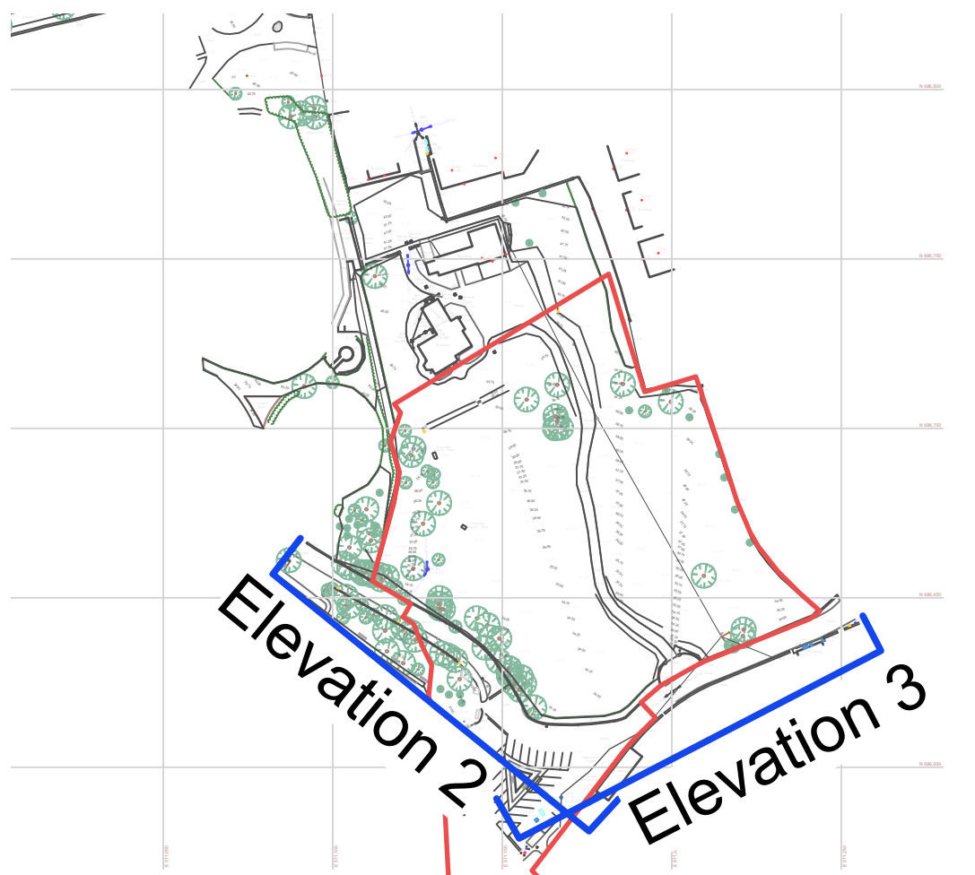
3 Key Plan Scale: 1:2000
